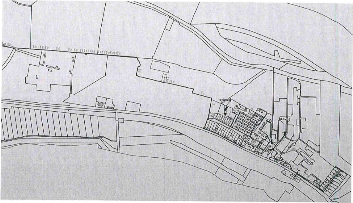
Melléklet: Almásfüzitő ivóvízhálózat helyszínrajz részlet
